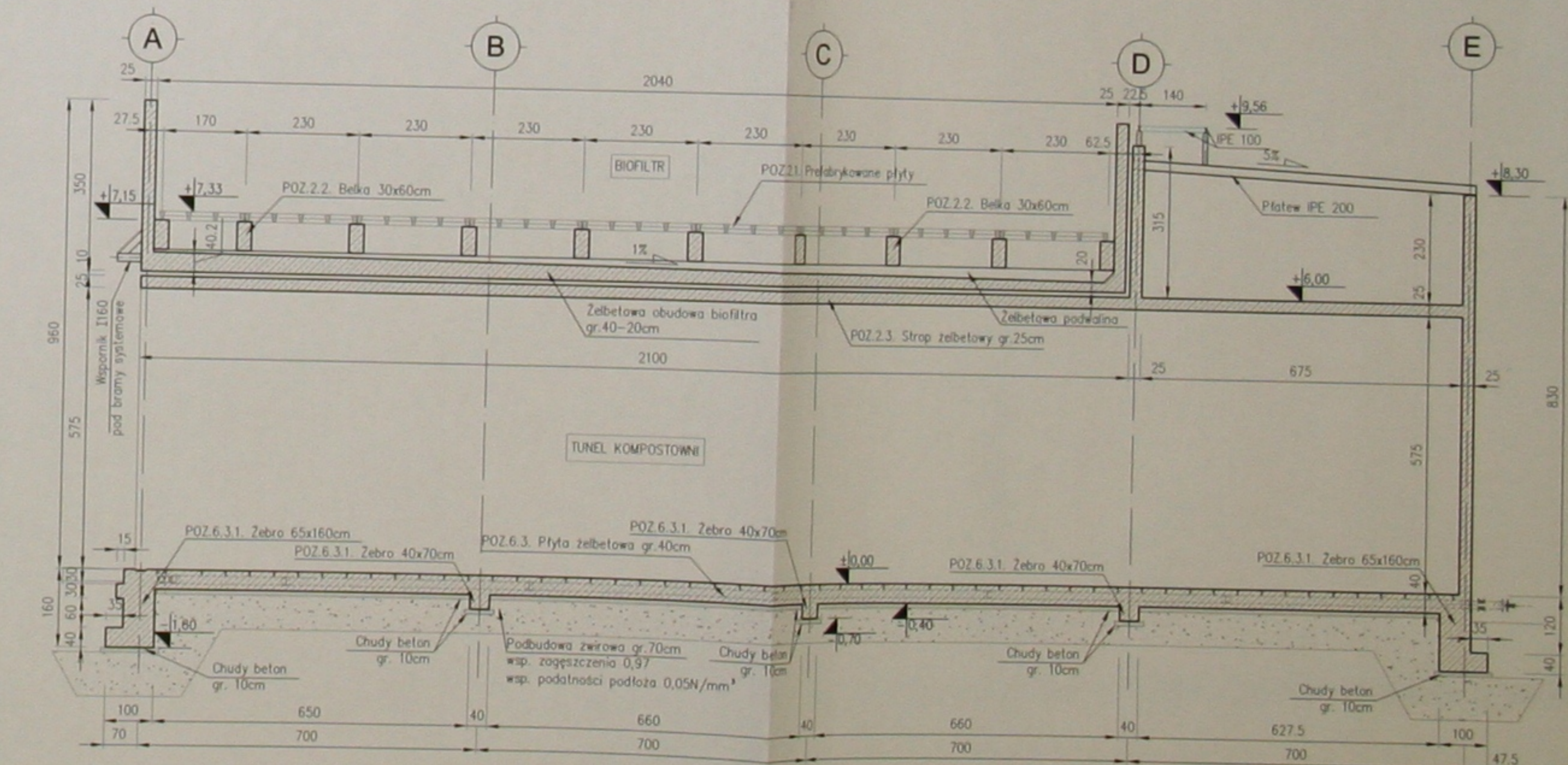
PRZĘKRÓJ PODŁUŻNY B-B
