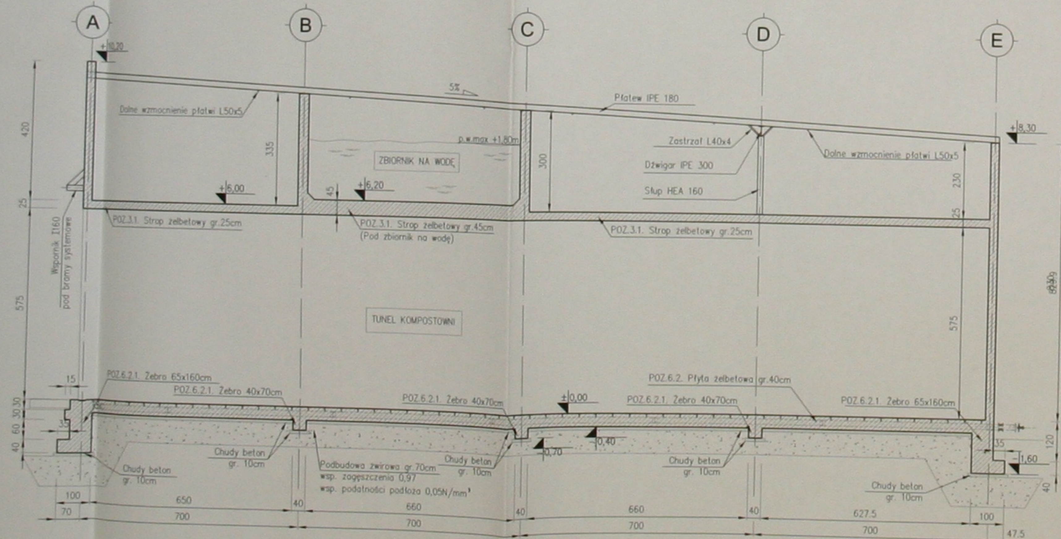
PRZĘKRÓJ PODŁUŻNY C-C
