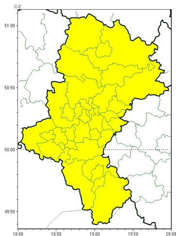
Opady marznące
